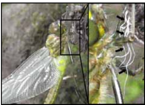
図 2 羽化の過程。右は黒枠の拡大。矢印はクチクラの脱皮を指す。
